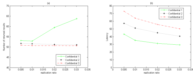
Fig. 6. DQ(f)+: Confidential Parameter impact
