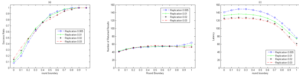
Fig. 2. Rounding Boundary impact to DQ
